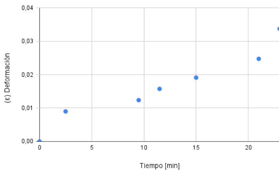
Figura 3: Gráfica del ensayo de termofluencia del aluminio ER4043
