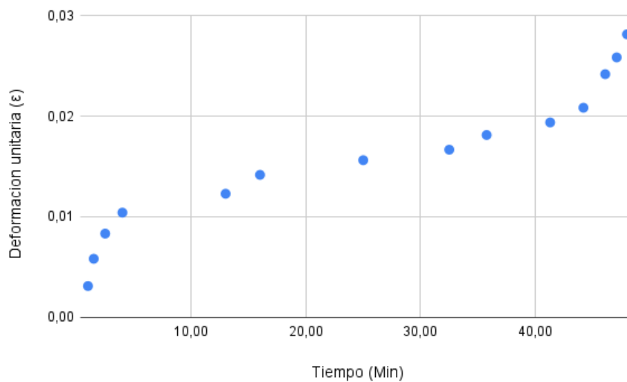
Figura 4: Gráfica del ensayo de termofluencia del acero AISI/SAE 1045.
