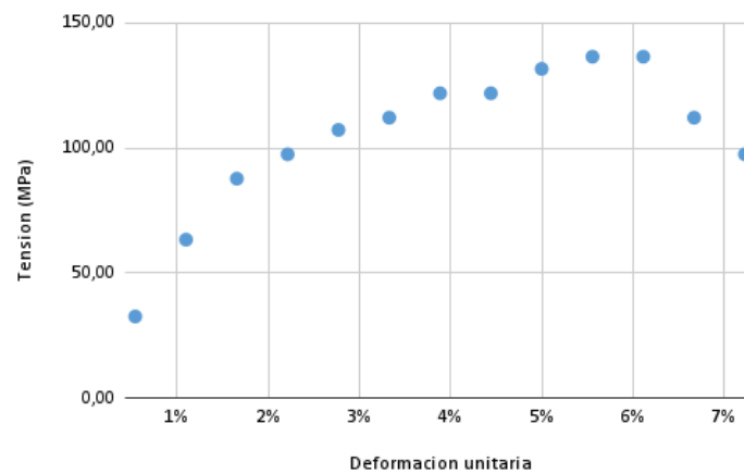
(b) Gráfica del ensayo de tracción del aluminio ER4043 ensayo 2.
