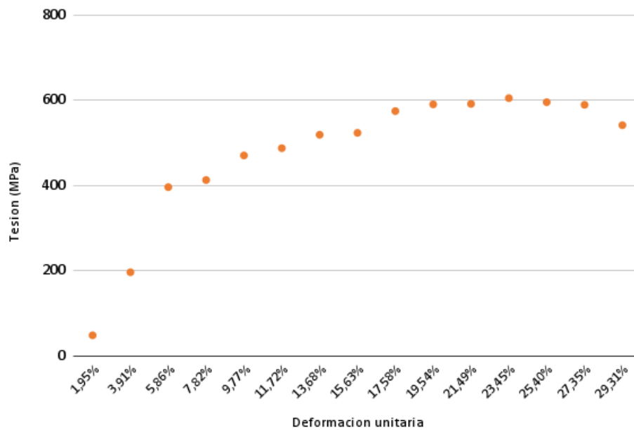
Figura 2: Gráfica del ensayo de tracción del 1045 SAE/AISI
