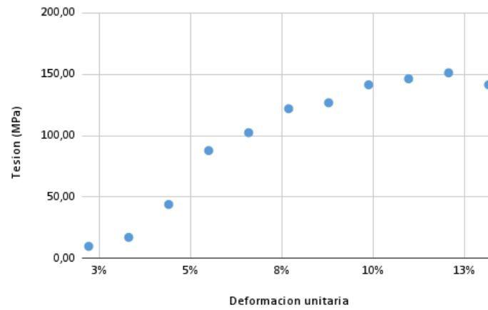
(a) Gráfica del ensayo de tracción del aluminio ER4043 ensayo 1.
